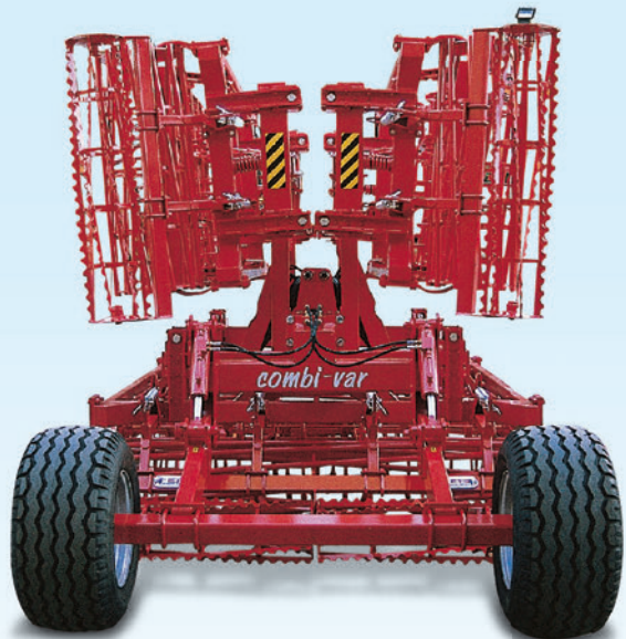
Macchina chiusa per trasporto su strada Closed machine pulling transport on the road
